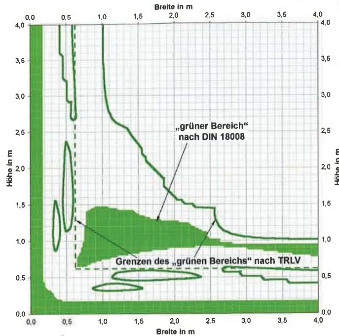
02: Bemessungsdiagramm für VSG-Glasaufbau 44/12/4/12/44, bei \pm 0,8 \text{ kN/m}^2 Windlast und 0,5 \text{ kN/m} Holmlast in 1 m Höhe über der Glasunterkante.
